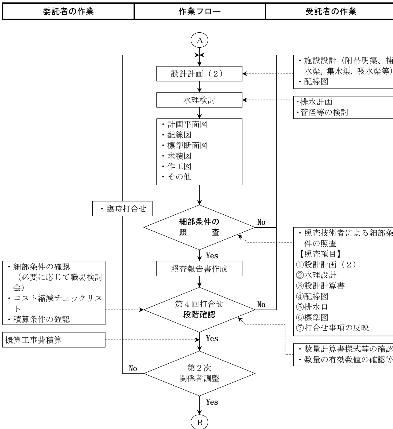
付表-1 実施設計照査フロー
